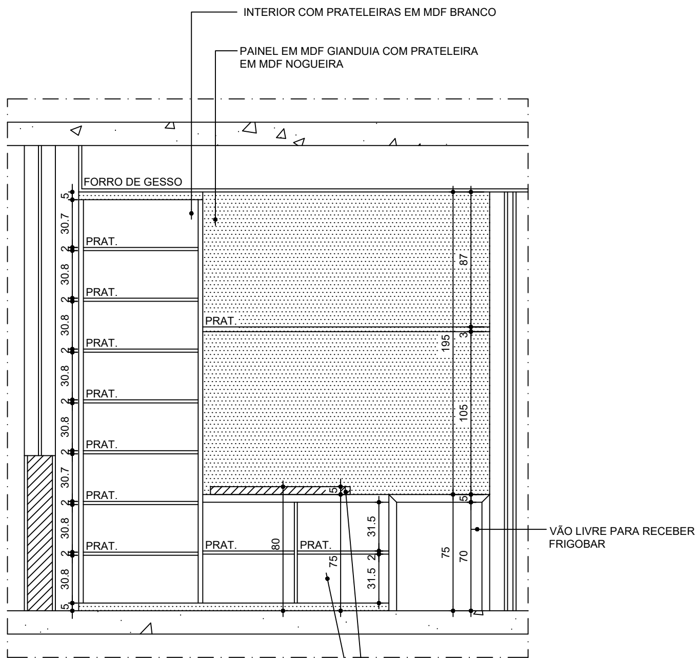
CORTE BB - INTERIOR DO ARMÁRIO ESCALA 1/25
