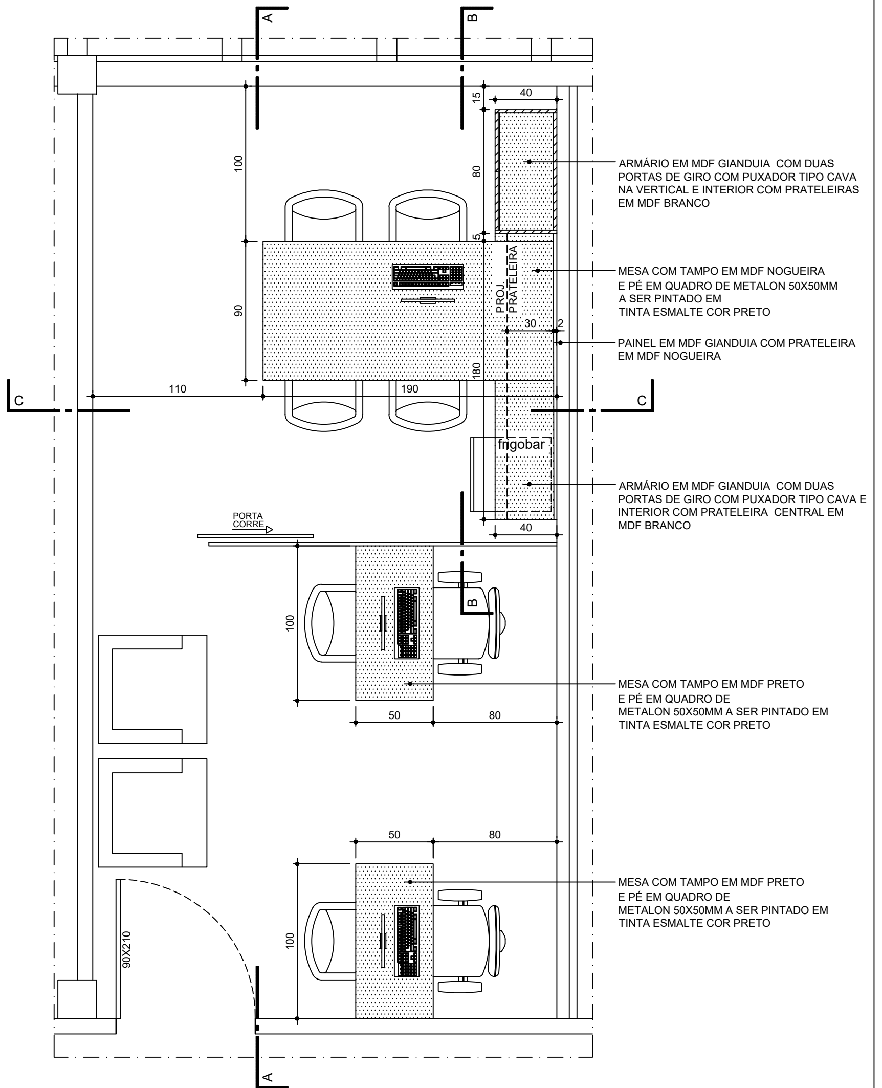
○ PLANTA GABINETE 01 ESCALA 1/25
